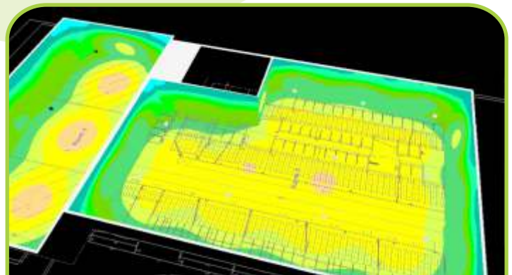
Lichtsimation Visualisierung der Beleuchtung
